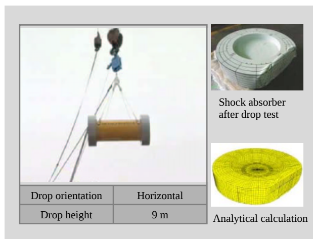
Fig. 6—1/3 Scale-model Drop Test Results.
