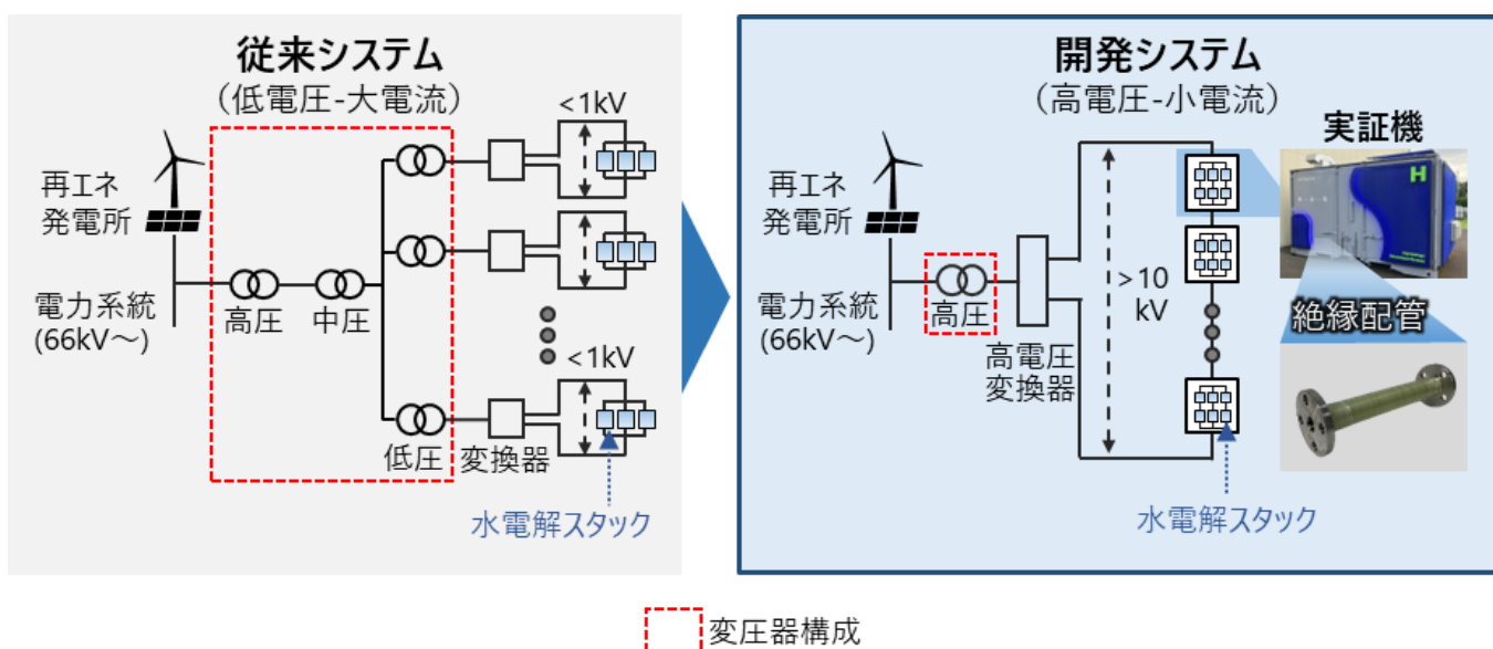
図1 従来の水電解システムと開発システムの比較
