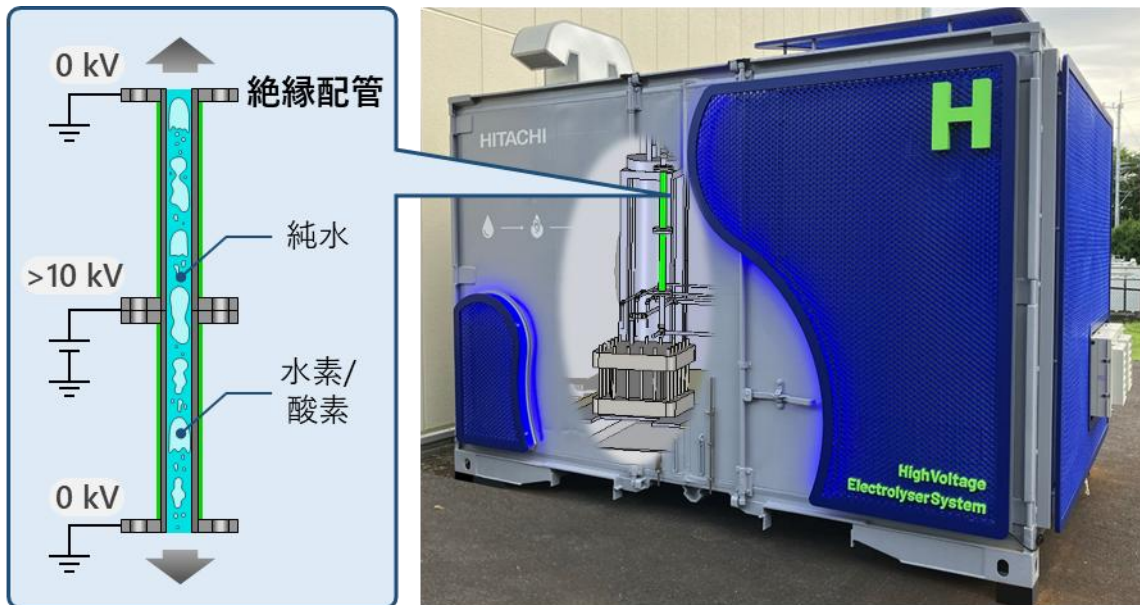
図 2 今回開発した絶縁配管の詳細イメージ
